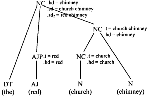
[그림 5] 두 개의 패턴부열을 가진 노드
