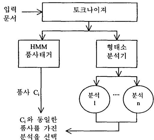
[그림 2] 형태소분석기의 구성도
