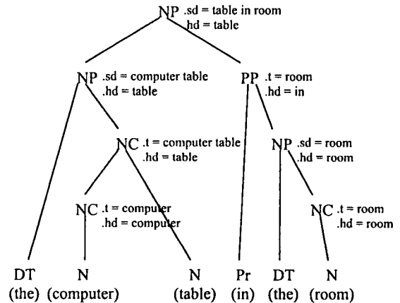
[그림 4] 전치사구 포함 명사구에 대한 구문트리 및 속성값
