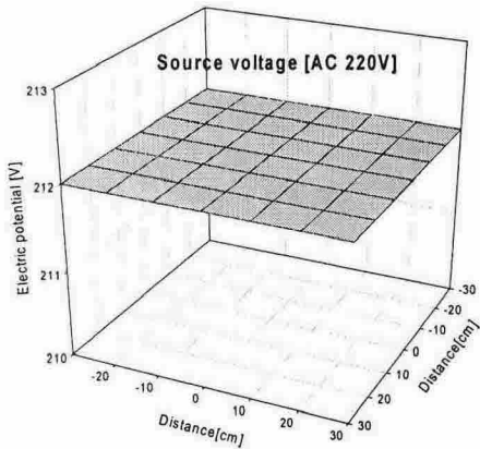
그림 8. case 3에 의한 전위 ( 금속제 욕조 )
