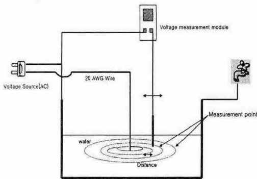
그림 2. 금속재 욕조 실험장치
