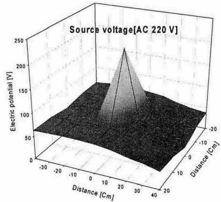
그림 7. case 2에 의한 전위 ( 아크릴욕조 )
