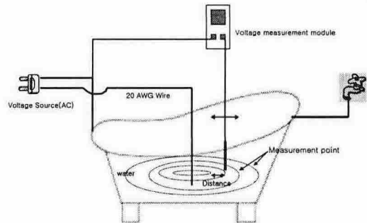
그림 3. 아크릴 욕조 실험장치
