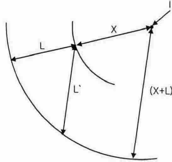
그림 1. 수중 전류원 (무한원점에 접지극이 있는 경우)
