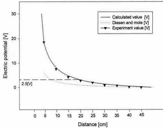
그림 10. 상용전원 220 [V]에서 거리에 대한 전위 (금속재 욕조)
