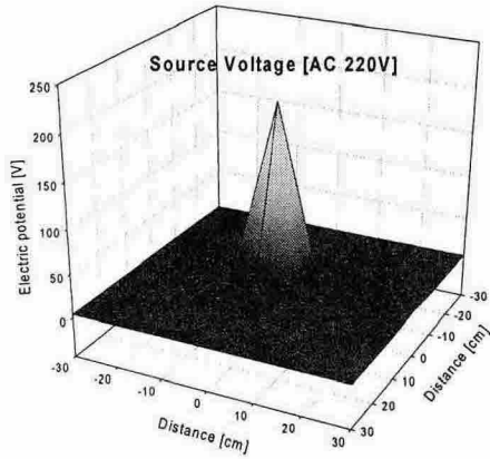
그림 4. case 1에 의한 전위 ( 금속제 욕조 )
