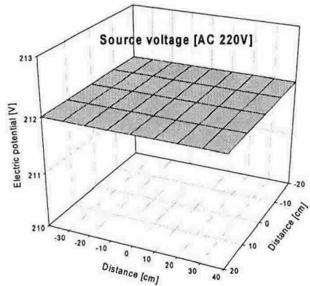
그림 9. case 3에 의한 전위 ( 아크릴욕조 )
