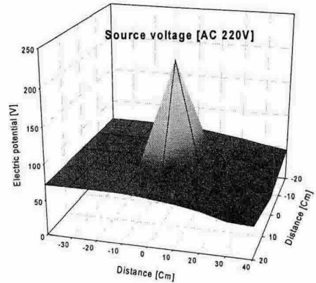
그림 5. case 1에 의한 전위 ( 아크릴욕조 )
