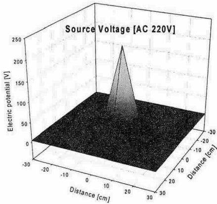
그림 6. case 2에 의한 전위 ( 금속제 욕조 )
