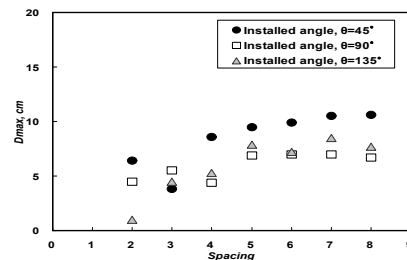
그림 6 수제설치간격에 따른 최대퇴적고
