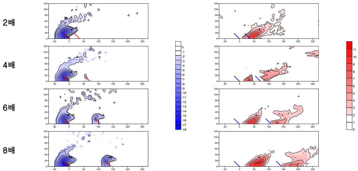
그림 4 수제 설치간격에 따른 하향수제 주변 세굴 및 퇴적(2배~8배)
