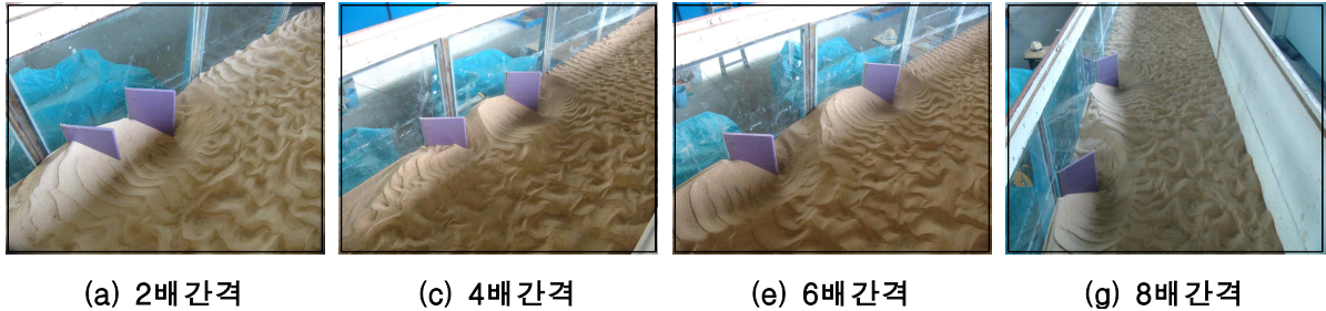
그림 3 수제 설치간격에 따른 수제 주변 세굴실험사진
