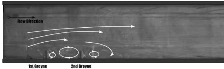
그림 1 군수제 주변 흐름특성개요도(자연공생하천구조물설계기술개발, 2010)
