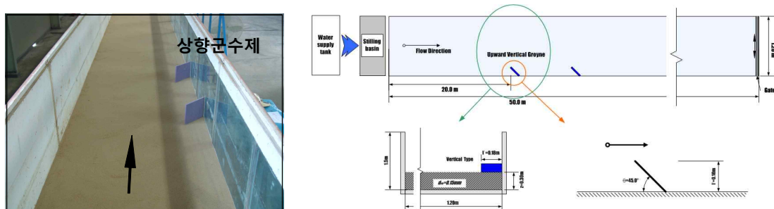
그림 2 실험수로 및 수제제원
