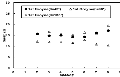
그림 7 설치각에 따른 비교(1st groyne)
