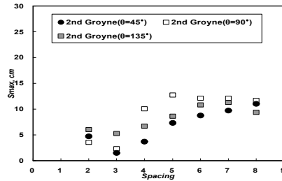
그림 8 설치각에 따른 비교(2nd groyne)
