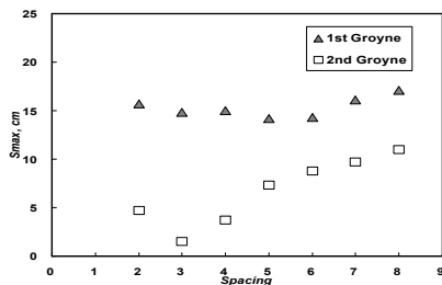
그림 5 수제설치간격에 따른 최대세굴심
