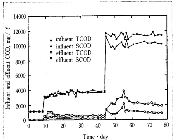
그림 1. Effect of organic loading rate on COD variation
