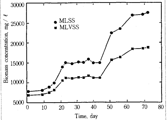
그림 4. Relationship between MLSS and MLVSS.
