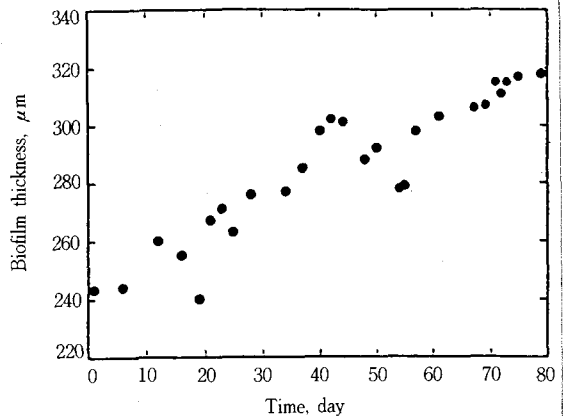
그림 5. Effect of organic loading rate on biofilm thickness.
