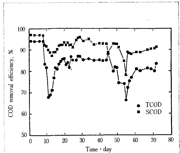
그림 2. Effect of organic loading rate on COD removal efficiency.
