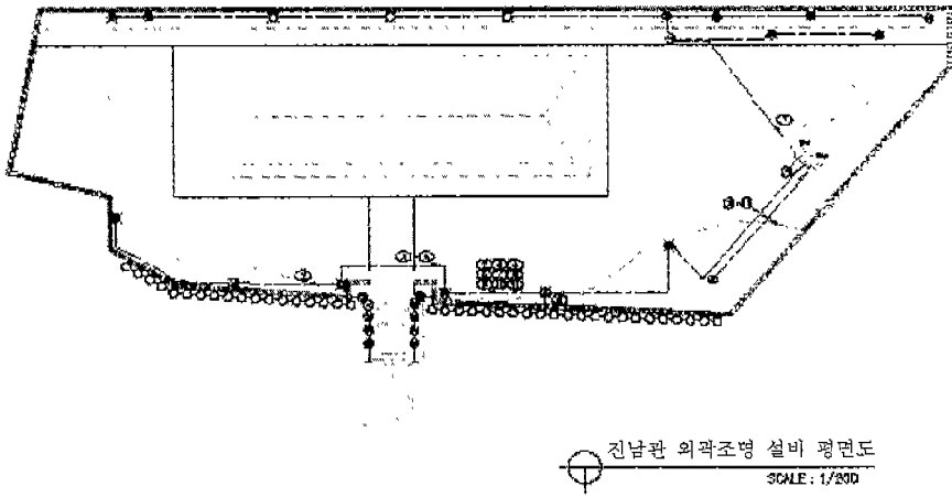
그림 8 진남관 본관건물과 외벽에 대한 등기구 배치도
