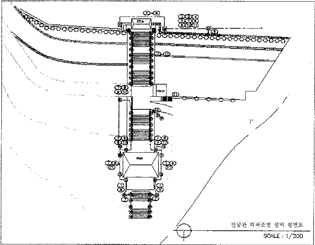
그림 10 계단 및 망해루 부분에 대한 조명설비 평면도
