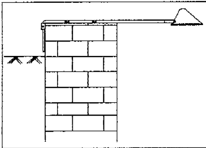
그림 6 진남관 문화재 관리사무실 외벽에 대한 등기구설치 방법
