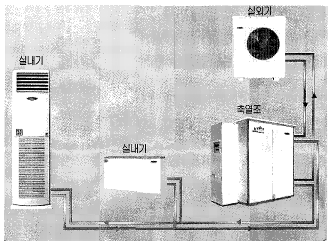
〈그림 4〉 소형 축냉식 냉방시스템 구성도
