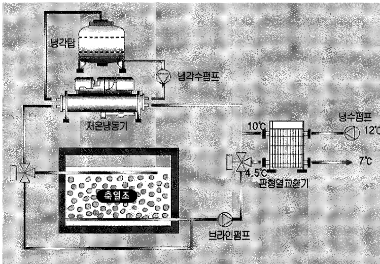
〈그림 3〉 축냉식 냉방설비 구성도
