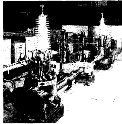
〈그림 6〉 고온초전도케이블 시스템 및 단말(도쿄전력)
