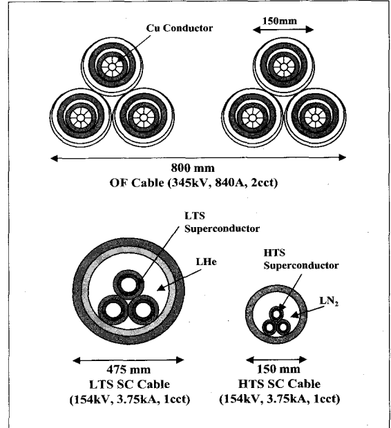
〈그림 3〉 1GVA용량의 케이블 크기 비교
