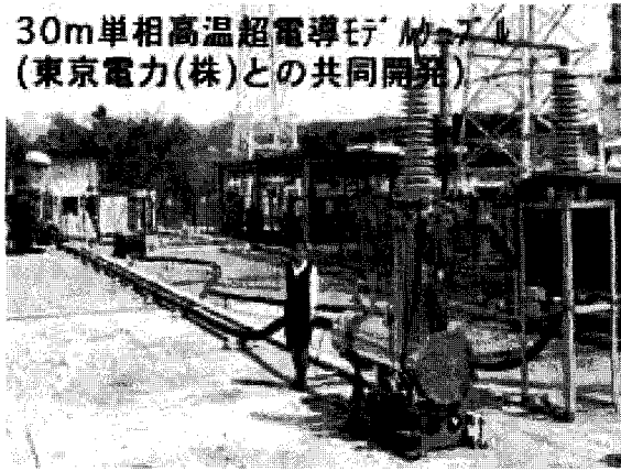
〈그림 6〉 고온초전도케이블 시스템 및 단말(도쿄전력)
