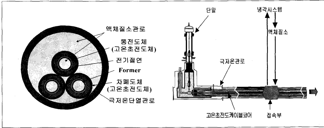
〈그림 2〉 고온초전도송전케이블의 단면구조 및 시스템 구성도
