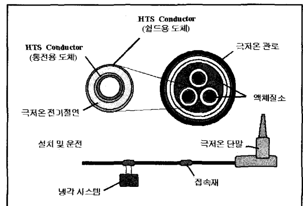
〈그림 5〉 초전도케이블 개발을 위한 주요 요소기술
