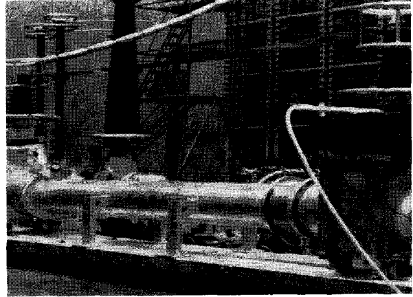
〈그림 7〉 154kV 800MVA급 극저온 저항케이블 송전시스템
