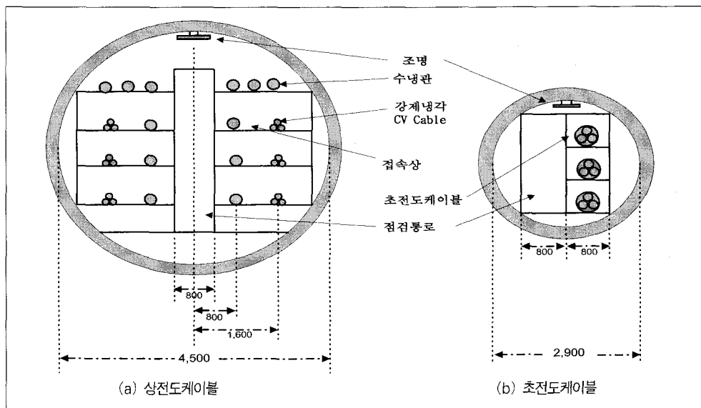
〈그림 4〉 전력구 규모의 비교
