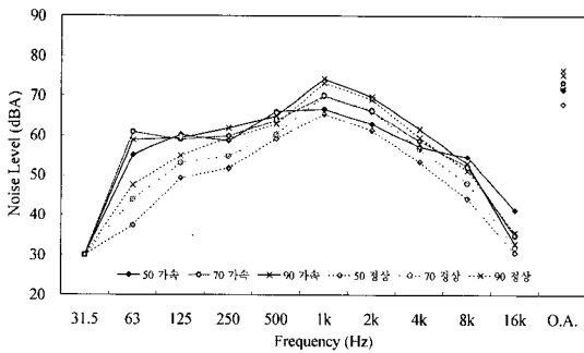
그림 4 Pass-by noise spectra of typical passenger vehicle(Verna)
