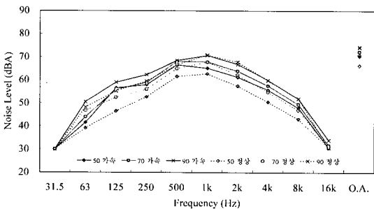
그림 5 Pass-by noise spectra of typical light goods vehicle(Santafe)
