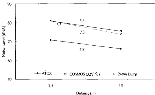
그림 8 Attenuation due to distance
