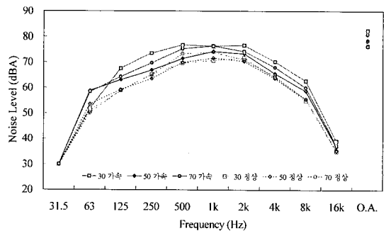
그림 7 Pass-by noise spectra of typical heavy omnibus(Gran Bird)
