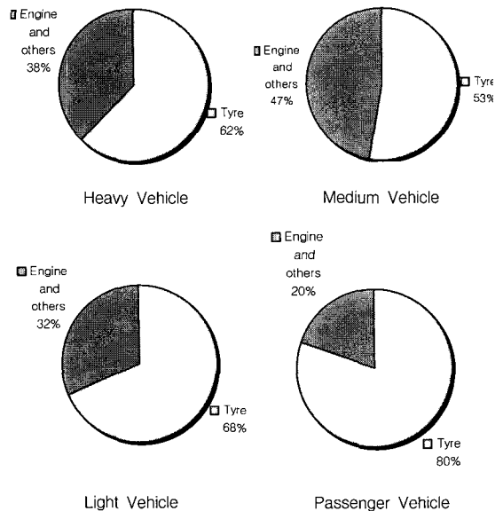
그림 9 Contribution ratio of individual noise source at pass-by
