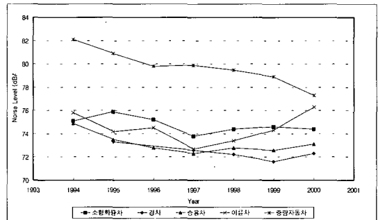
그림 1 Acceleration noise of vehicle by year
