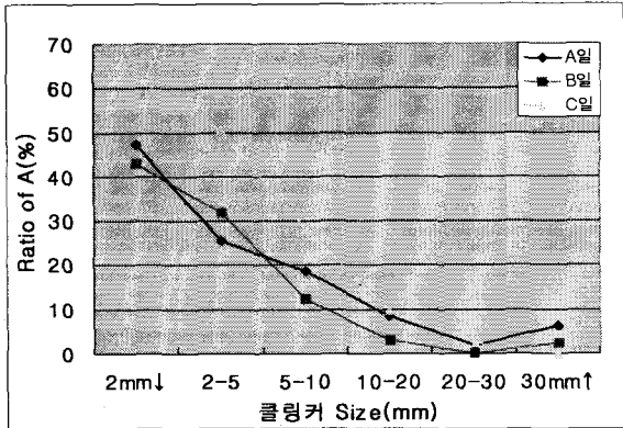
<그림 5> 클링커 nodule size별 냉각지수
