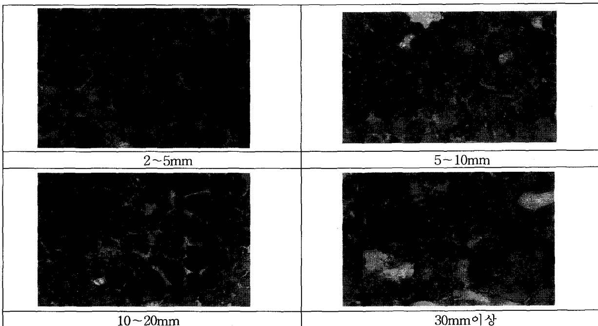
<그림 6> 클링커 nodule size별 광물조직 변화
