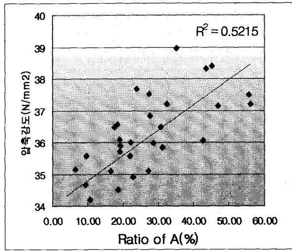
<그림 8> 평균화된 공장클링커의 냉각지수와 압축강도 관계
