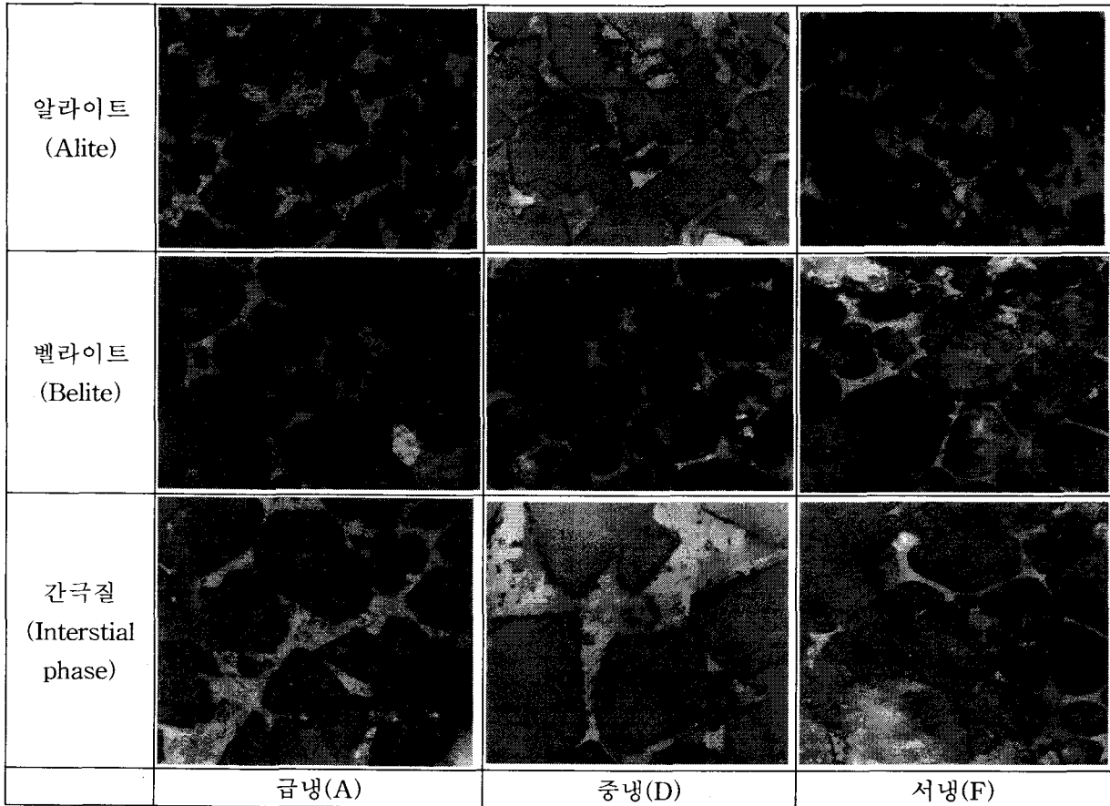
< 그림 2 > 냉각조건별 실험실적 제조 클링커의 미세조직
