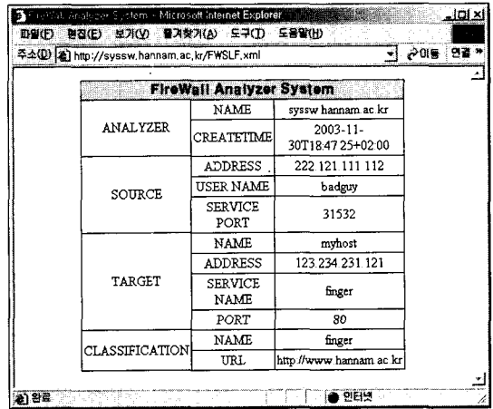
(그림 10) XSLT 적용 결과
