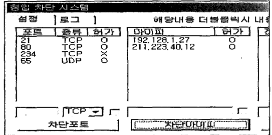
(그림 6) 필터링 설정
