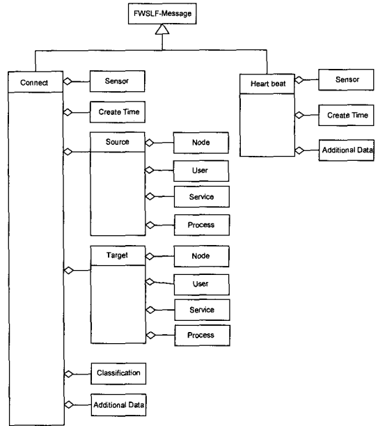
(그림 2) 침입차단 시스템 로그 포맷
