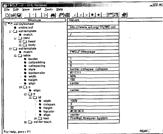
(그림 9) XML 문서에 대한 XSLT 문서
