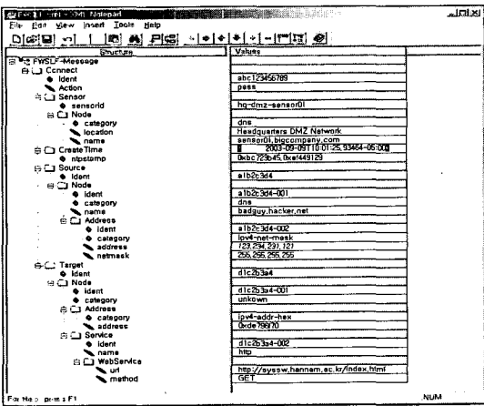
(그림 8) 침입차단 로그에 대한 XML 문서
