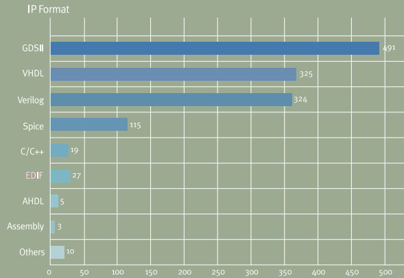
Format별 IP개수
