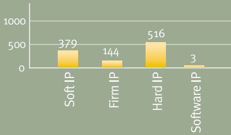
Type별 IP개수
