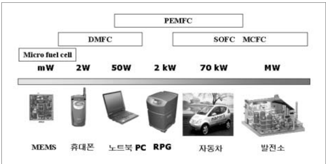
▲ 그림 3. 연료전지의 종류에 따른 활용분야
