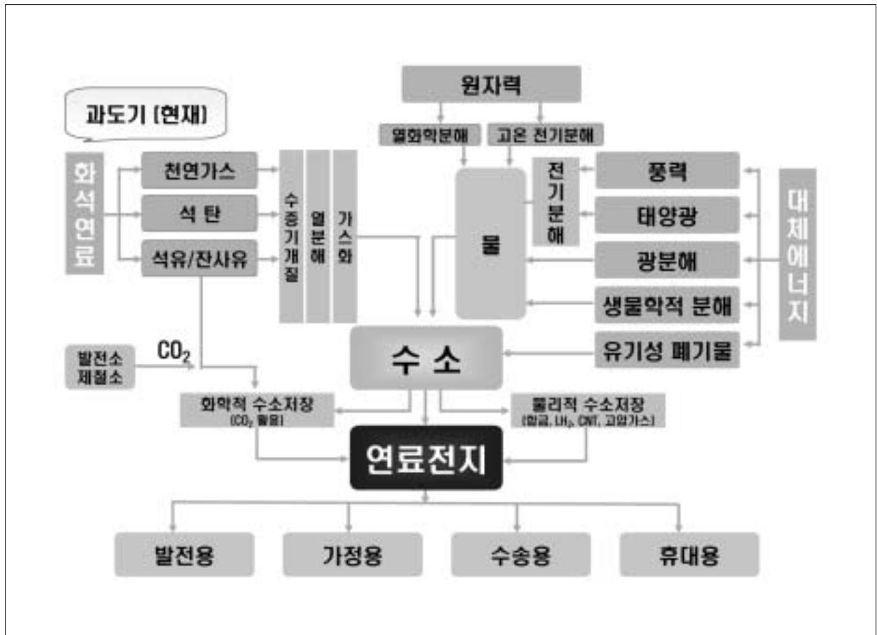
▲ 그림 1. 수소 제조기술 및 연료전지 기술의 계통도
