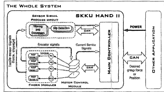
그림 6. SKKU hand II의 시스템 구성도. Fig. 6. System schematic of SKKU hand II.
