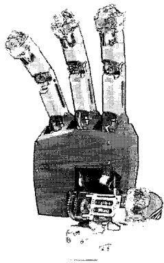
그림 1. KKU hand II와 촉각센서. Fig. 1. SKKU hand II with tactile sensor.
