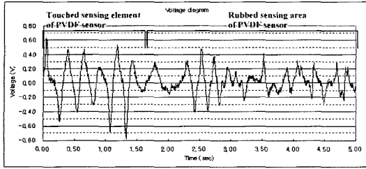
그림 11. 접촉 및 미끌림에 대한 단일 신호 출력. Fig. 11. Signal output from touching and rubbing.
