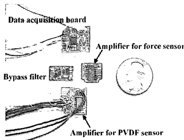
그림 10. 촉각 센서 시스템 구성. Fig. 10. Photograph of tactile sensing system.
