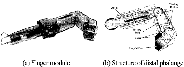
그림 2. 손가락 모듈. Fig. 2. Finger module.
