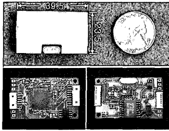
그림 5. 모터 제어 보드. Fig. 5. Motor control board.
