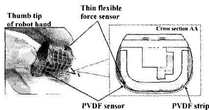
그림 9. 촉각 센서의 구조. Fig. 9. Structure of fingertip tactile sensor.
