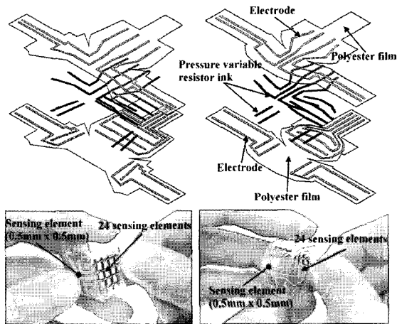
그림 8. 손가락 끝부분의 힘센서. Fig. 8. Fingertip force sensor.
