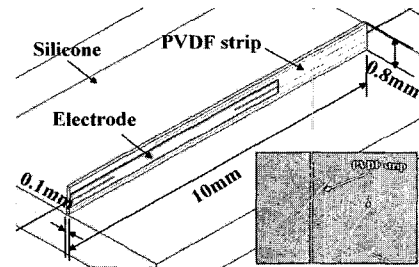
그림 7. PVDF 센서 도면 및 사진. Fig. 7. Schematic of PVDF sensor and photograph.
