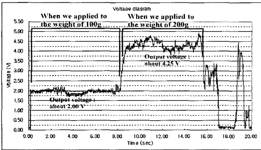
그림 13. 100g과 200g 추에 대한 응답 비교. Fig. 13. Response to the weight of 100g and 200g.
