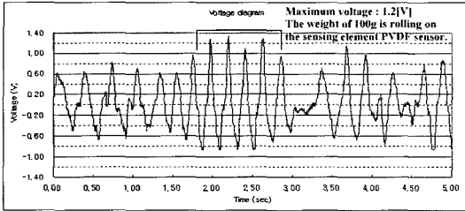
그림 12. 100g 추의 굴림에 대한 단일 신호 출력. Fig. 12. Signal output from rolling of 100g weight.
