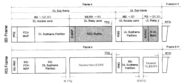
그림 8 Non-Transparent Frame Structure의 예
