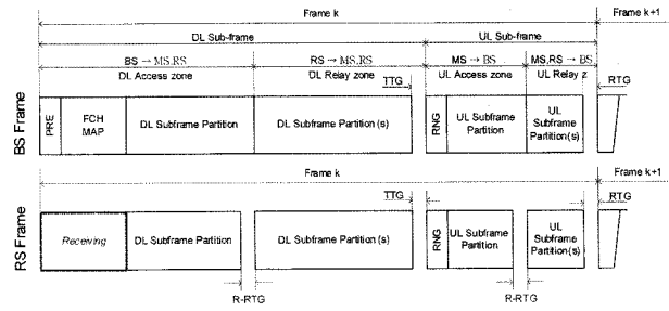
그림 7 Transparent Frame Structure의 예
