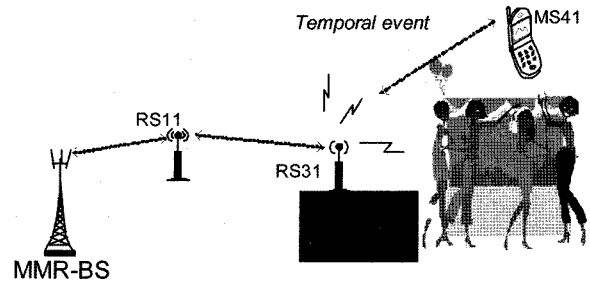
그림 4 Temporary Coverage RS Model
