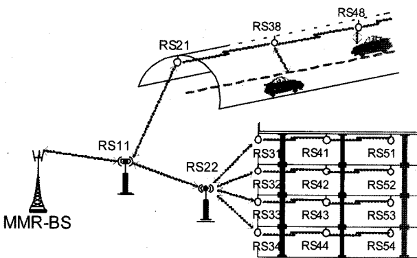
그림 3 In-Building Coverage RS Model
