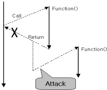
(그림 2) 버퍼 오버플로워 공격의 기본 개념
