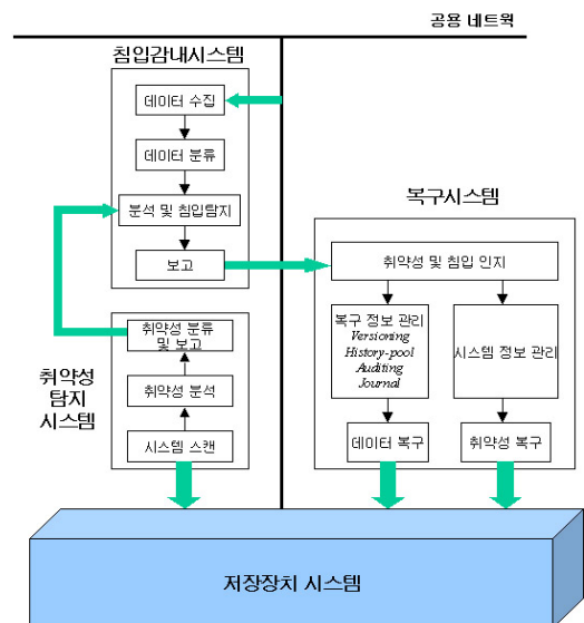
(그림 4) 안전한 저장장치시스템의 구성도
