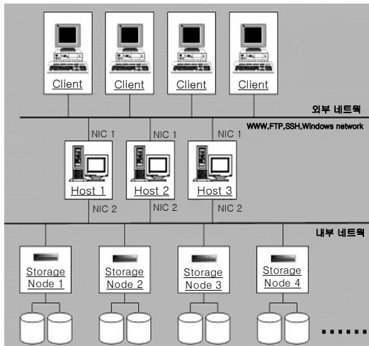
(그림 1) 저장장치시스템의 구성도
