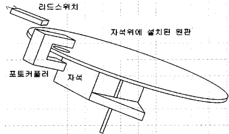
[그림 2] 디지털 펄스 수도계량기의 구성도
