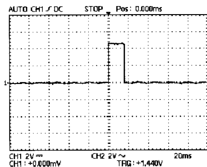
(b) 출력신호(OUT) 파형
