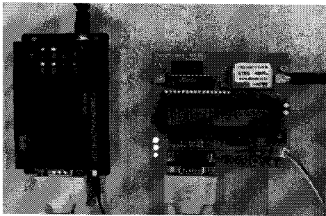
[그림 11] 개발한 중계기 외관
