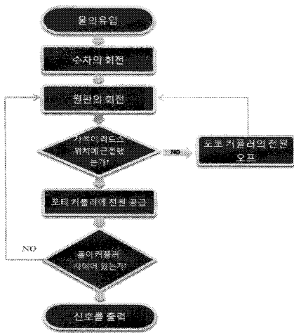
[그림 3] 펄스 수도 계량기의 작동
