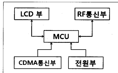
[그림 10] 중계기 구성
