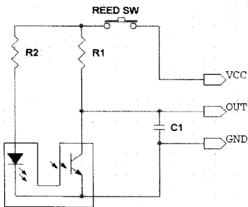
[그림 4] 디지털 펄스 수도 계량기 회로도
