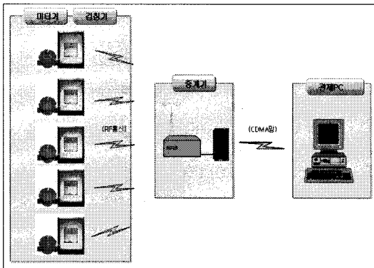
[그림 1] 상수도 원격검침 시스템의 구성
