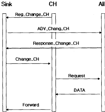
[그림 3] CH 재-선출 단계
