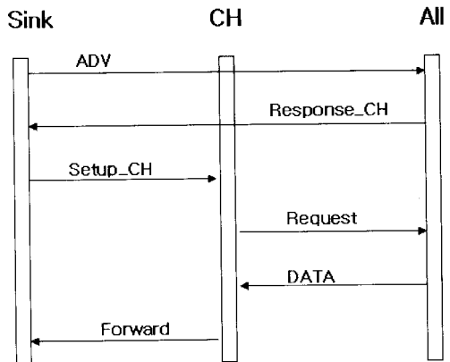
[그림 2] 초기 CH선출 단계
