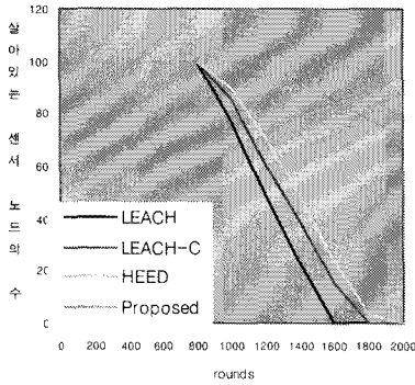
[그림 5] 노드 생존율 비교
