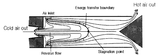
[그림 2] 볼텍스 튜브의 에너지 분리 원리 개략도
