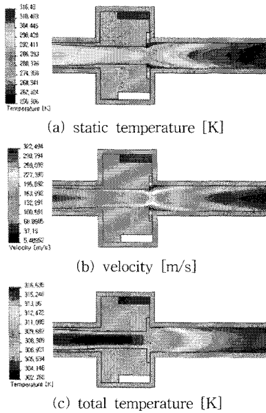
[그림 5] 볼텍스 발생기내의 온도 및 속도 분포 (Base model)
