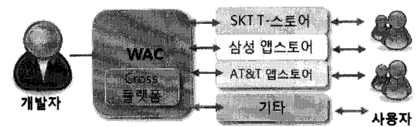
그림 2 WAC 기반 앱스토어 구조
