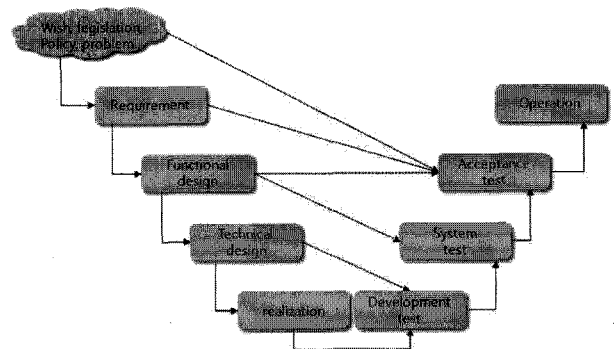
그림 3 V-모델과 테스팅
