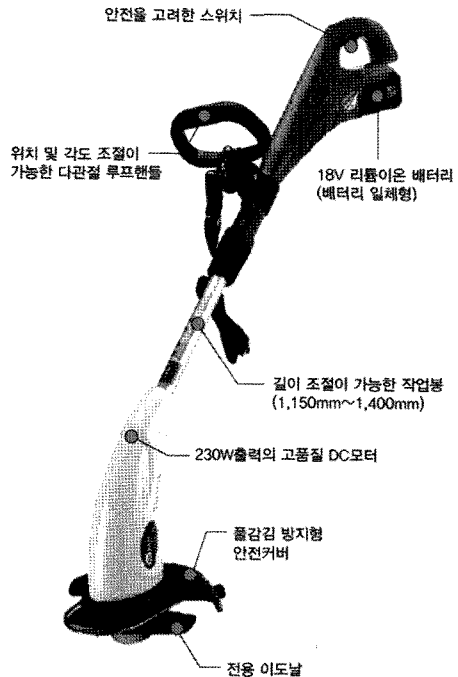
▲ 충전 예초기(KCB-180)
