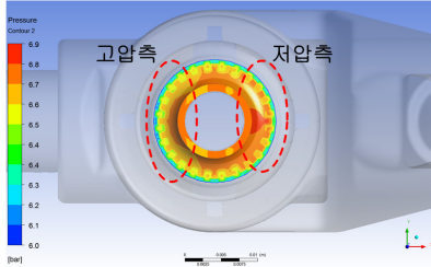
[그림 6] 디스크 상부 표면에서의 압력 분포 [Fig. 6] The pressure result in the upper surface of the disk
