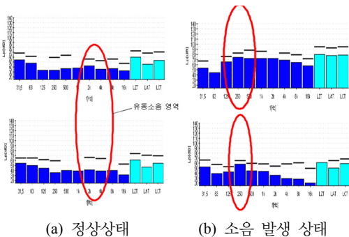
[그림 3] 아파트의 감압밸브 배관에 대한 음압 측정 결과 [Fig. 3] Results of noise measurements of piping system including the PRV in a apartment.
