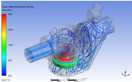
[그림 7] 감압 밸브 내부의 유동 패턴 [Fig. 7] The flow pattern of the pressure reducing valves
