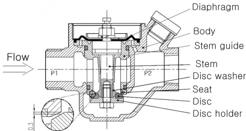
[그림 2] 감압밸브의 내부 구조도 [Fig. 2] The internal structure of the PRV.
