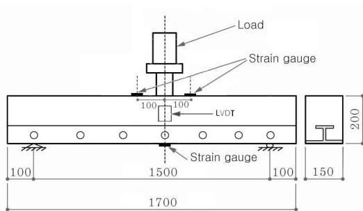
[그림 1] 합성보의 형상 및 실험장치[9]
