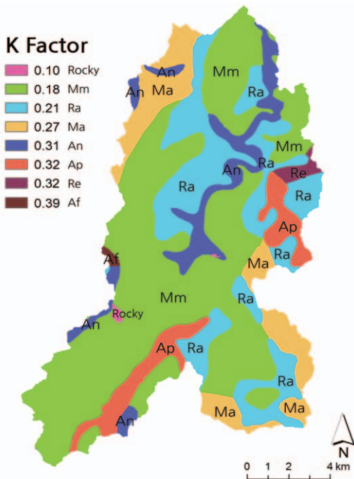
그림 4. 소옥천 유역의 토양침식인자(K)
