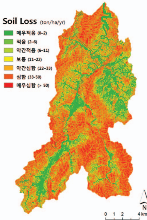
그림 8. 소옥천 유역의 토양유실 등급
