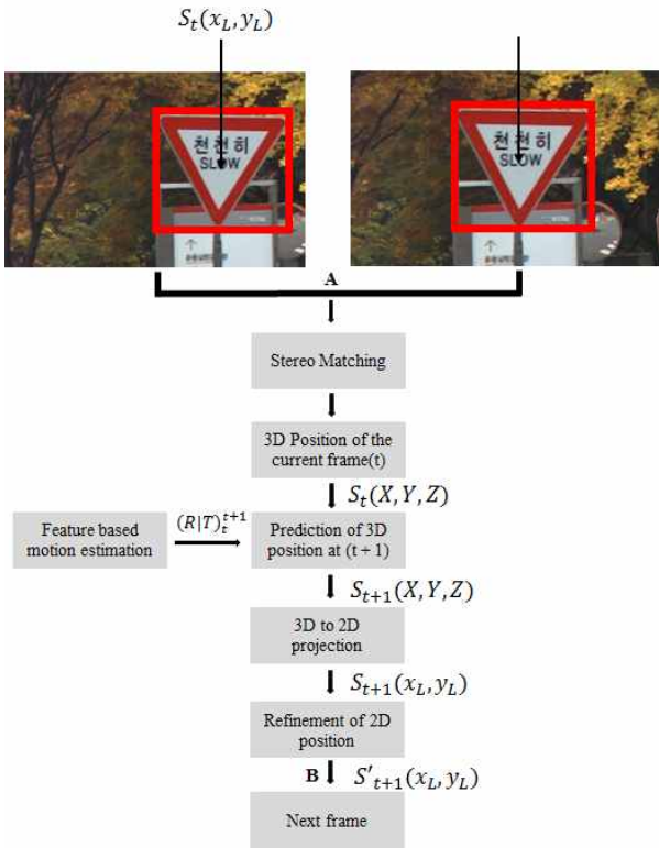
그림 6. 차량 모션과 스테레오 기반의 추적 알고리즘. Fig. 6. Sign tracking algorithm based on vehicle motion and stereo vision.
