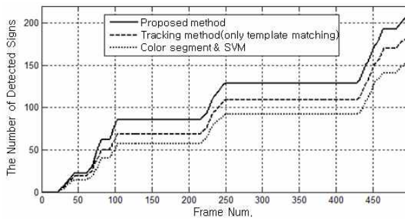
그림 11. 다양한 방법에 대한 표지판 검출수 그래프.
