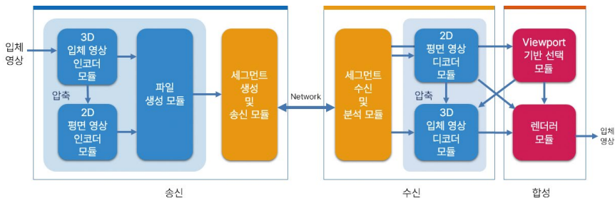
그림 4 입체영상 송수신 및 합성 기술 개념도
